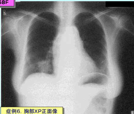
症例6. 胸部XP正面像
