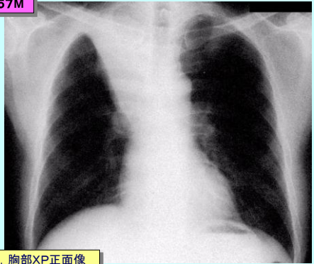
症例4. 胸部XP正面像
