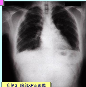
症例3. 胸部XP正面像
